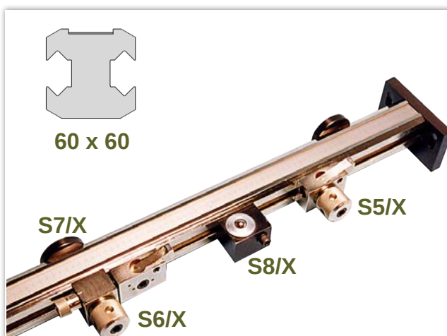
R30 RIFERIMENTO PER CESOIA REFERENCE FOR SHEAR
