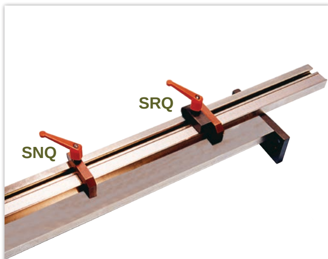
SQ SQUADRA PER CESOIA SQUARING ARM FOR SHEAR temprata ad induzione - induction hardened
